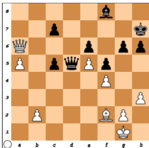
Diagram 3. Leon - Ebe na 32. a5
