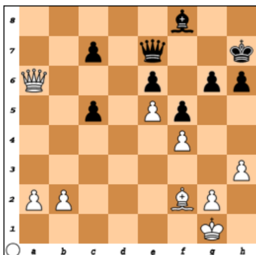
Diagram 2. Leon - Ebe na 30. Dxa6
