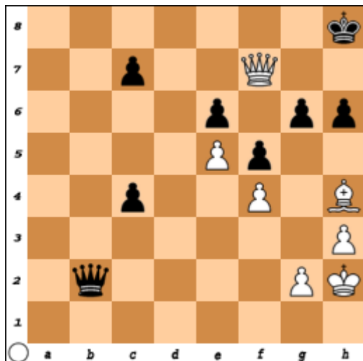
Diagram 5. Leon - Ebe na 37. Lh4
